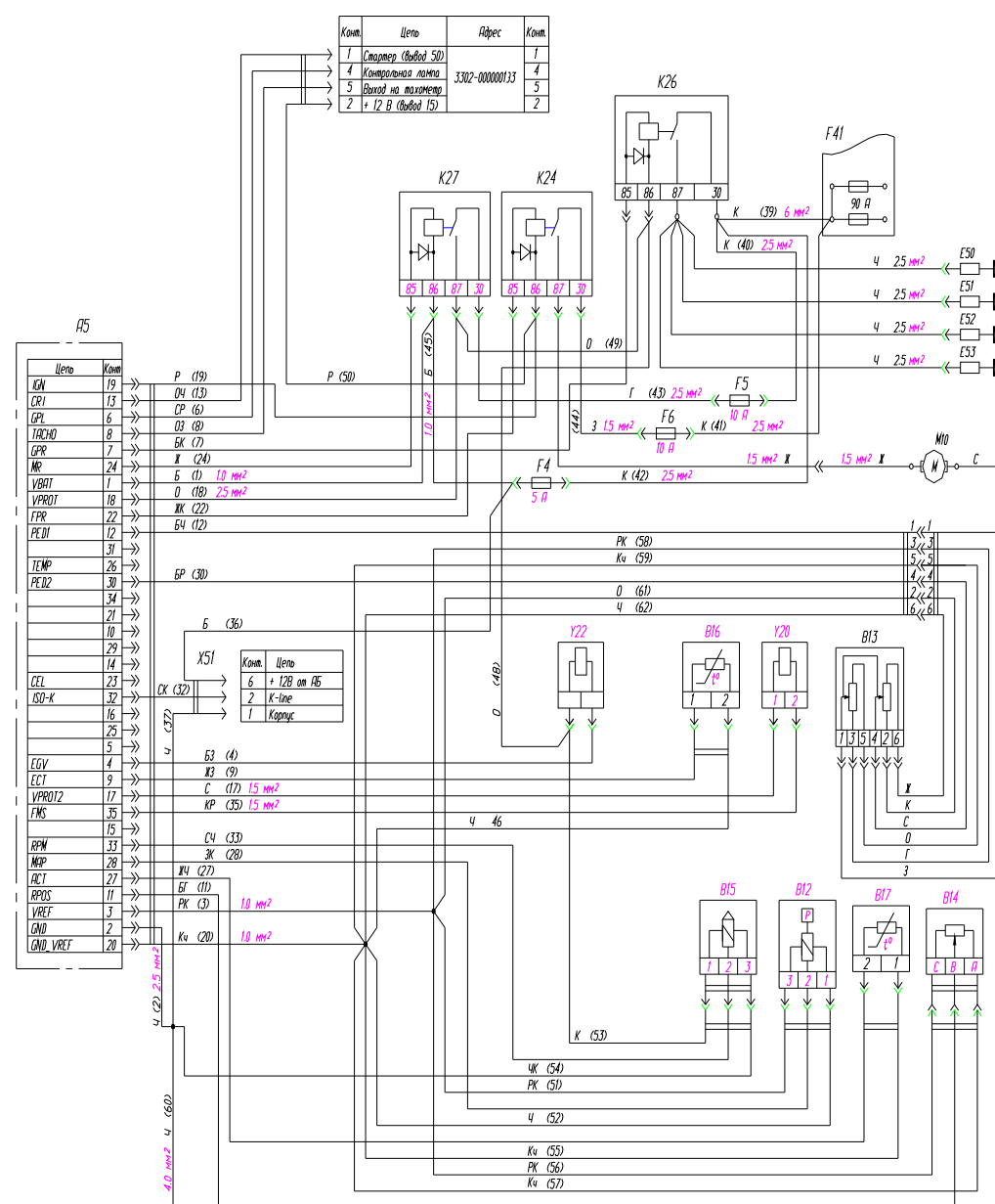
Схема системы управления двигателем
