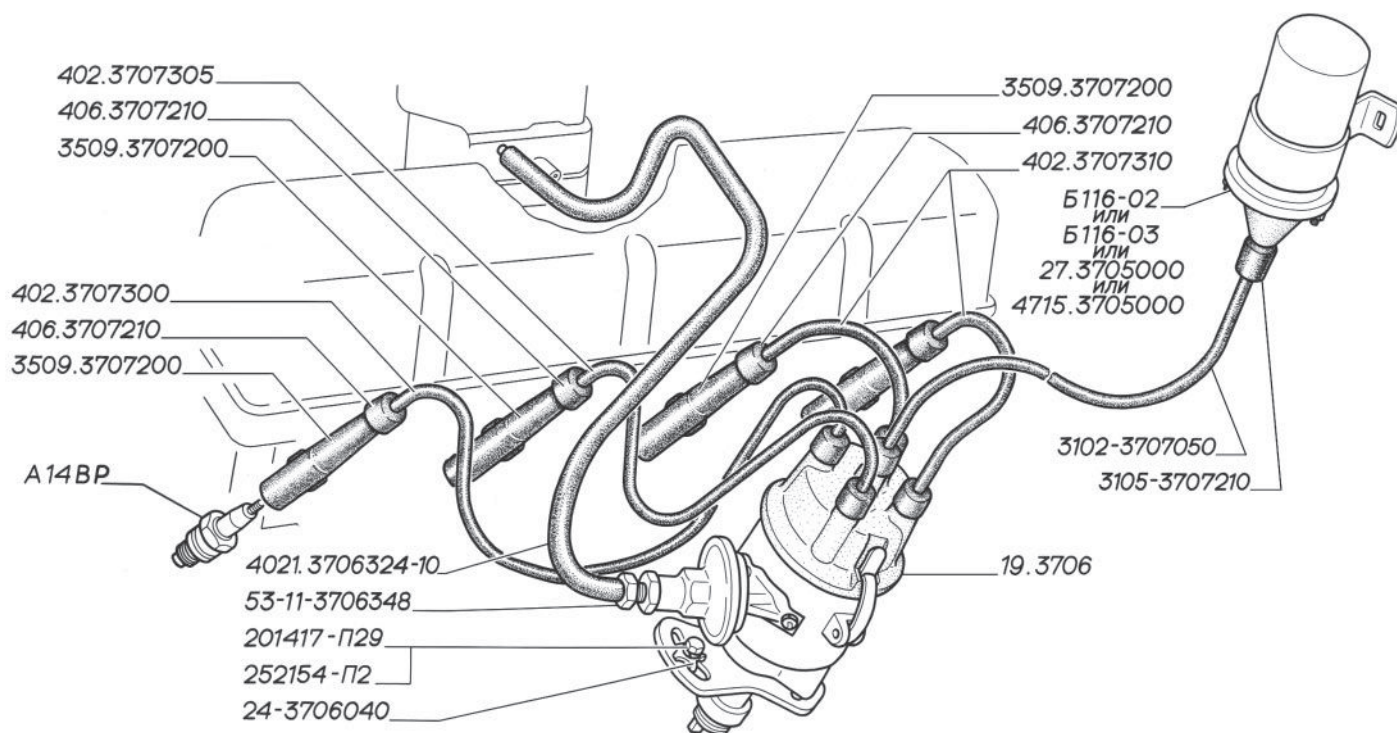
Рис. 75. Катушка зажигания, датчик-распределитель, провода и свечи двигателей ЗМЗ-402
