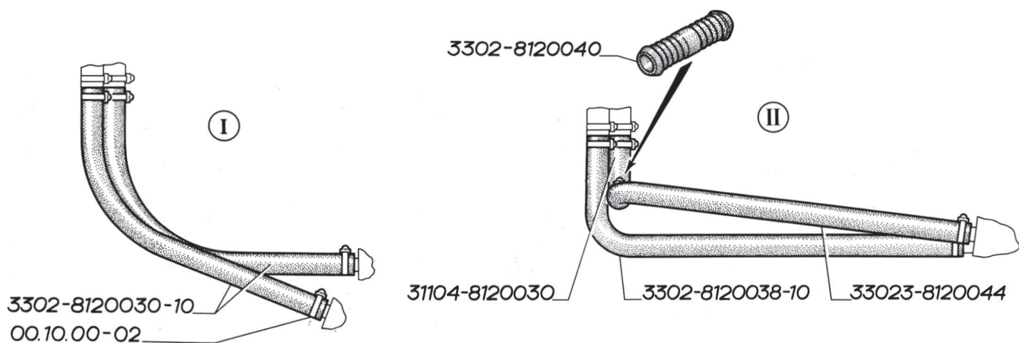
Рис. 125. Трубопроводы отопителя (для автомобилей выпуска с 2003 г.): I – для автомобилей с двигателем ЗМЗ-406; II – для автомобилей с двигателями ЗМЗ-402 и УМЗ-4215
