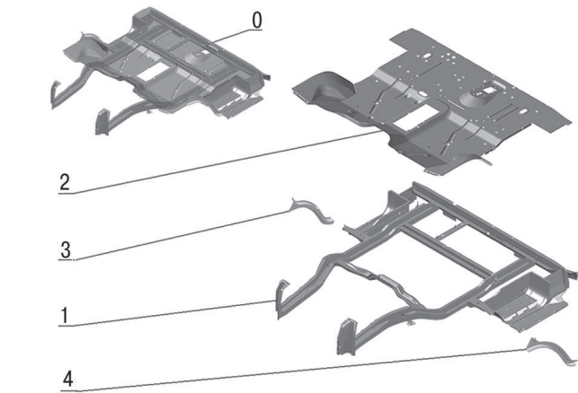
Рис. 6. Каркас с полом передний (2705-5101012)
