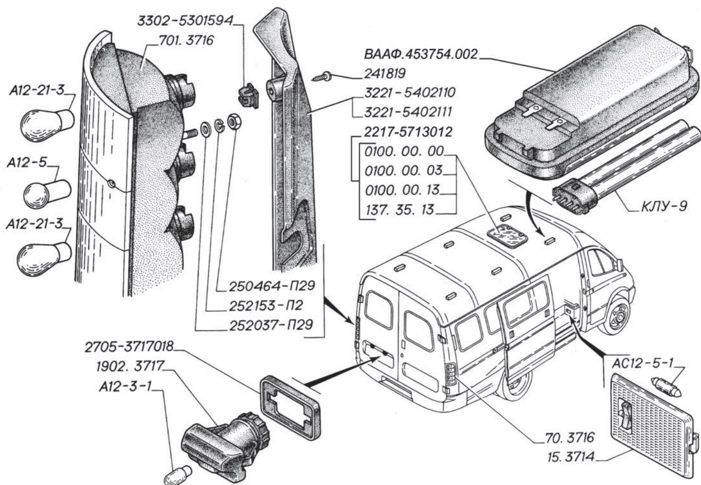
Рис. 14. Люк крыши, плафоны пассажирского салона, задние фонари
