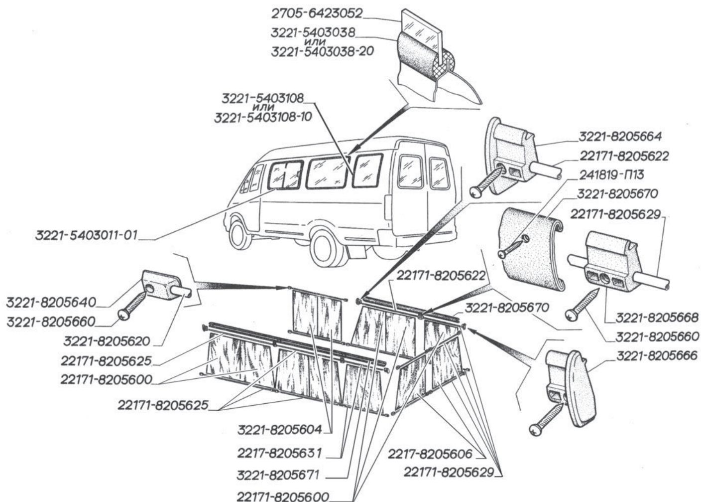
Рис. 21. Окна боковины, шторы
