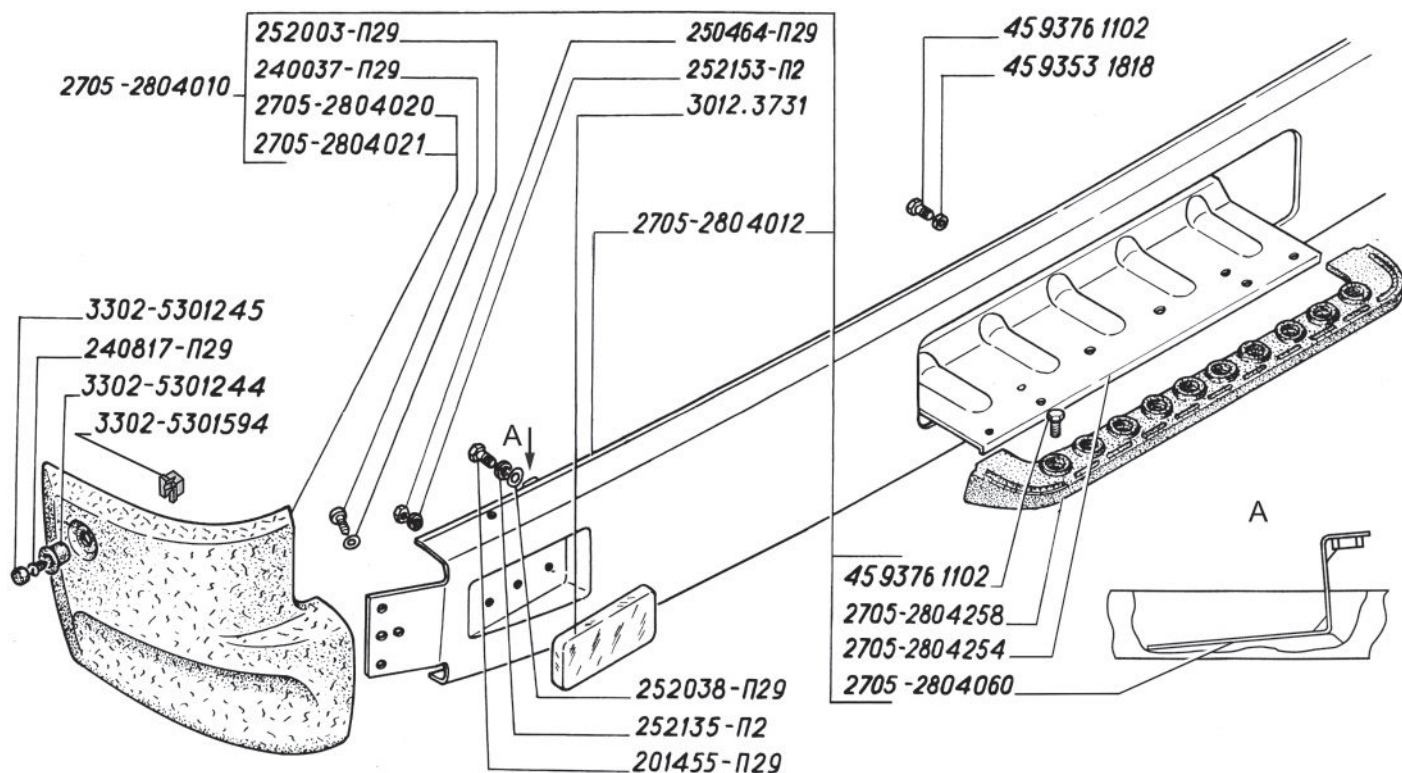
Рис. 2. Бумпер задний и световозвращатель (для автомобилей выпуска до 2003 г.)
