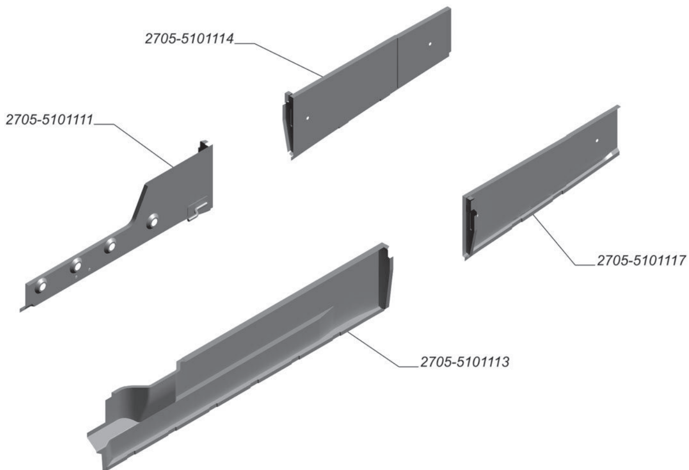
Рис. 92. Лонжероны фургона
