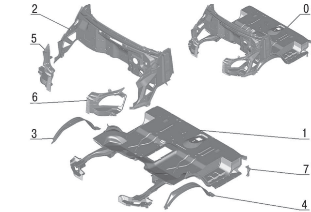
Рис. 161. Пол автобуса передний (3221-5101010-10)
