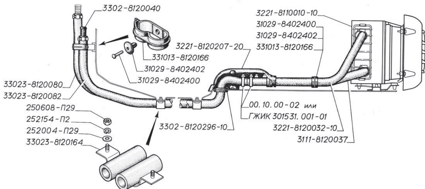
Рис. 31. Трубопроводы заднего отопителя автобусов
