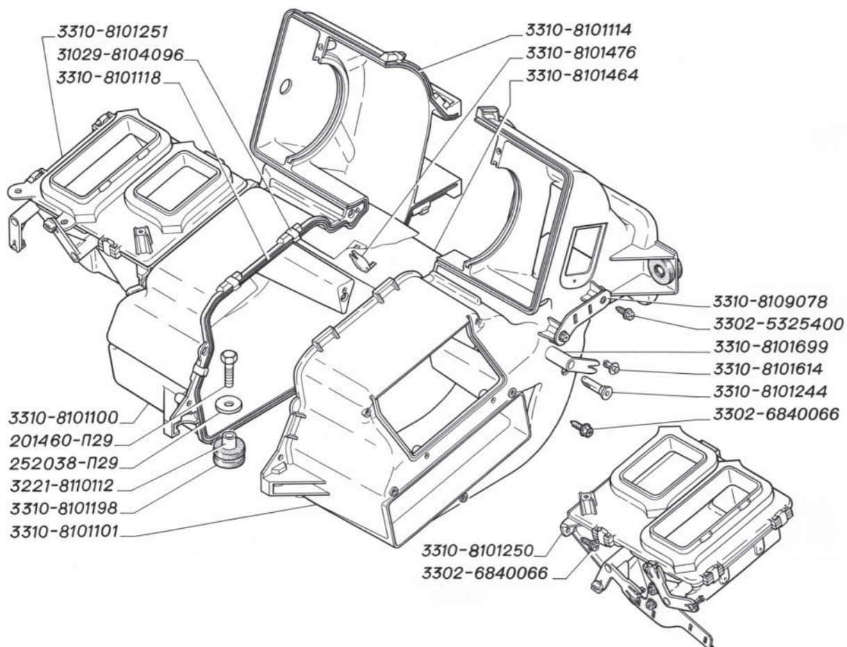
Рис. 124. Детали корпуса отопителя (для автомобилей выпуска с 2003 г.)
