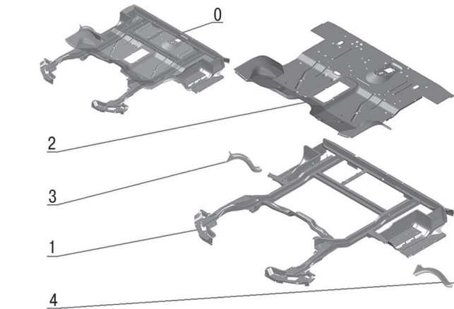
Рис. 7. Каркас с полом передний (3221-5101012-10)
