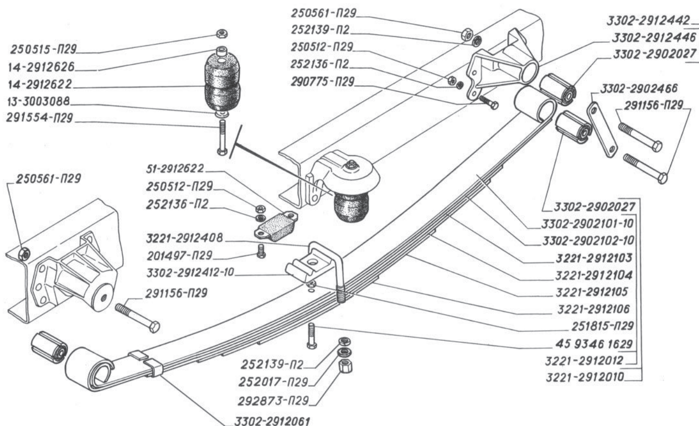
Рис. 3. Рессора задняя, крепление задних рессор
