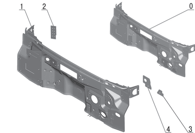
Рис. 160. Щиток передка с боковыми панелями передка (2217-5301080)
