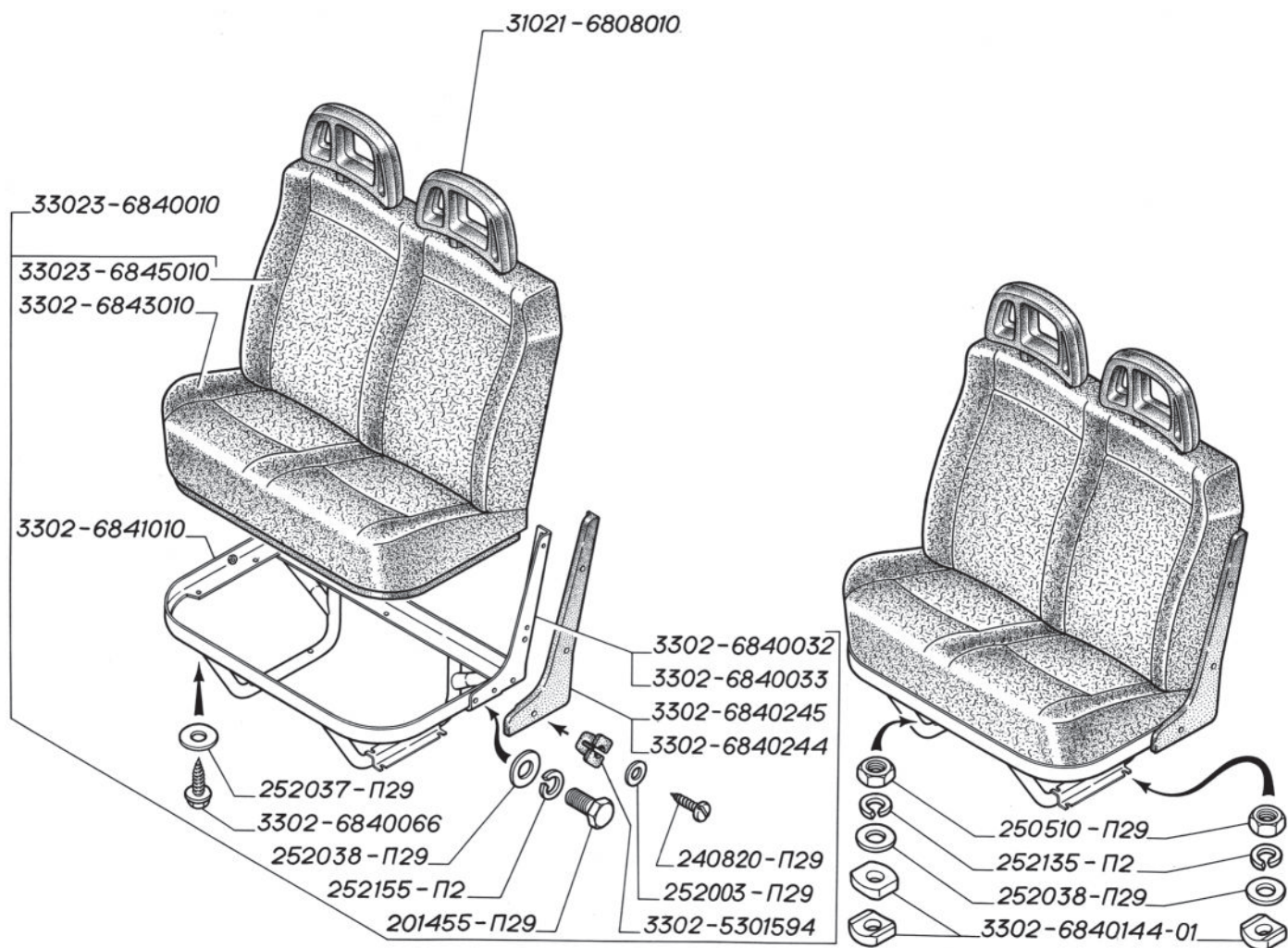
Рис. 115. Двухместное сиденье кабины
