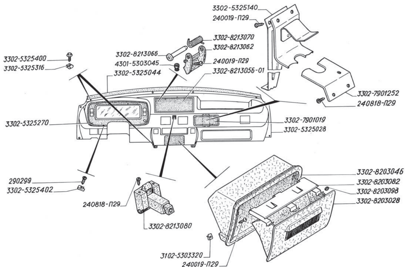
Рис. 99. Панель приборов (для автомобилей выпуска до 2003 г.)
