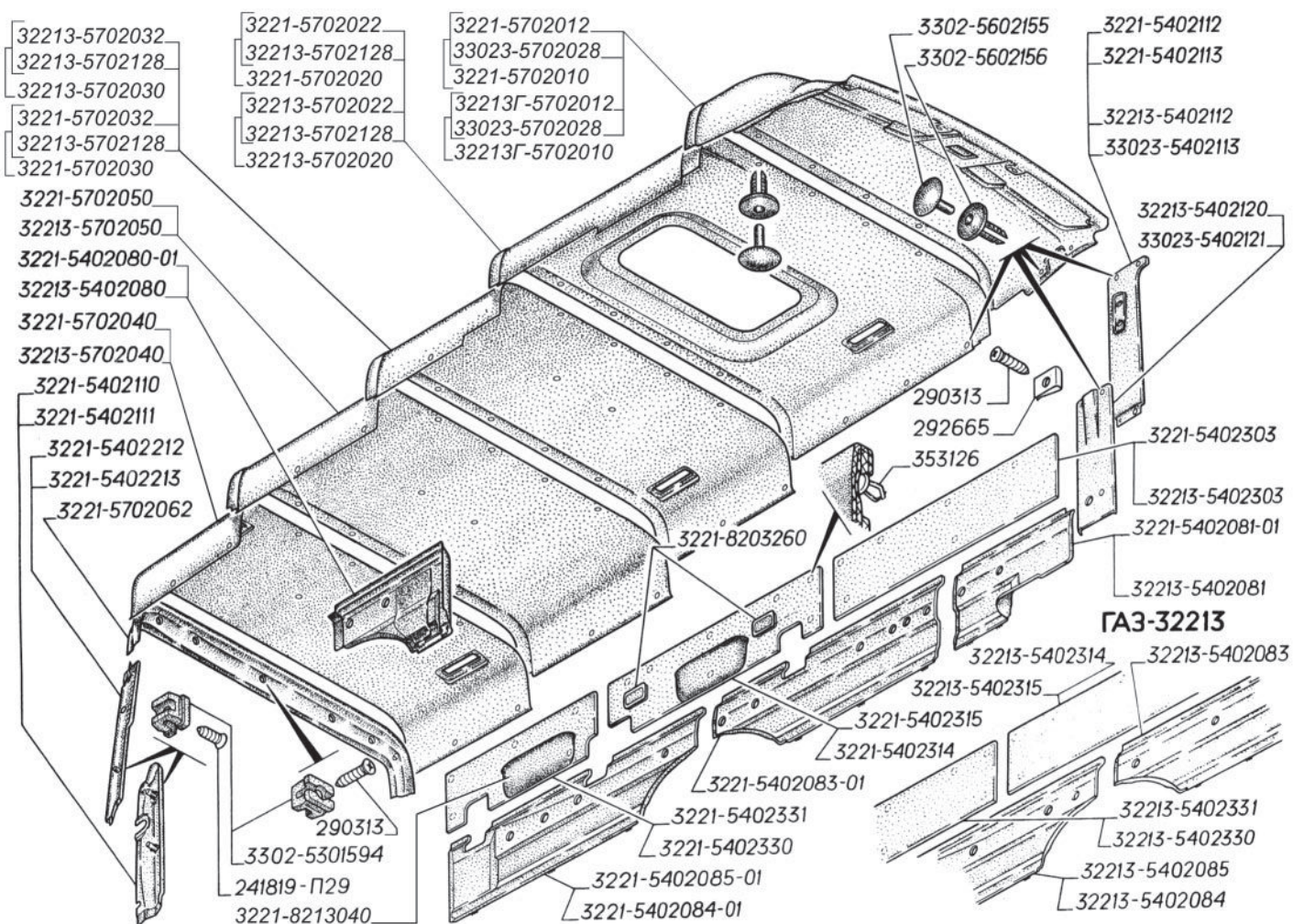
Рис. 17. Обивка пассажирского салона автобусов ГАЗ-3221 и ГАЗ-32213
