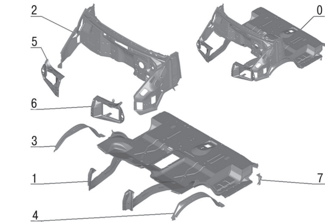
Рис. 162. Пол фургона передний (2705-5101010)
