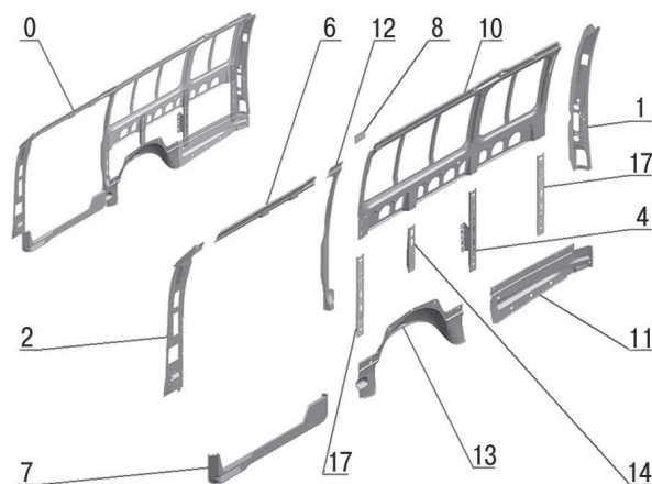
Рис. 135. Каркас правой боковины (2705-5401050)
