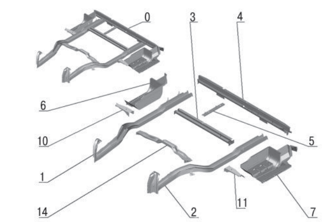
Рис. 12. Каркас пола (2705-5101014)
