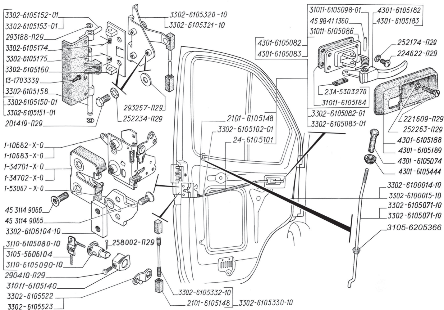
Рис. 107. Замок и ручки передних дверей (для автомобилей выпуска с февраля 2004 г.)
