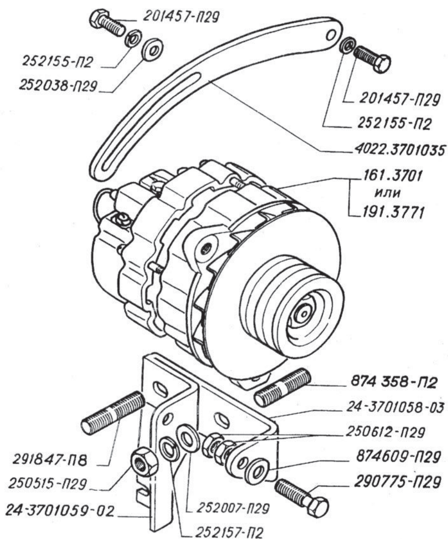
Рис. 73. Генератор двигателей 3М3-402
