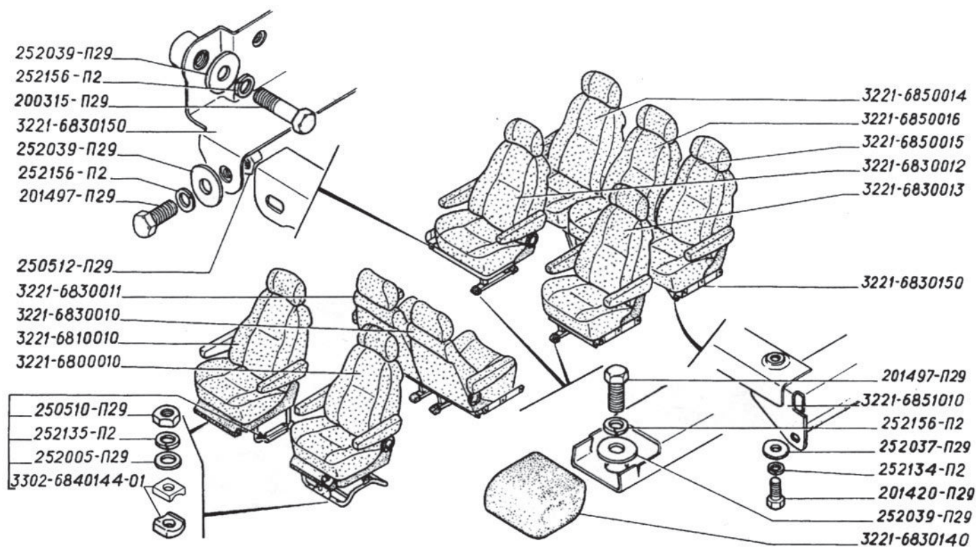
Рис. 22. Установка сидений автобуса ГАЗ-3221
