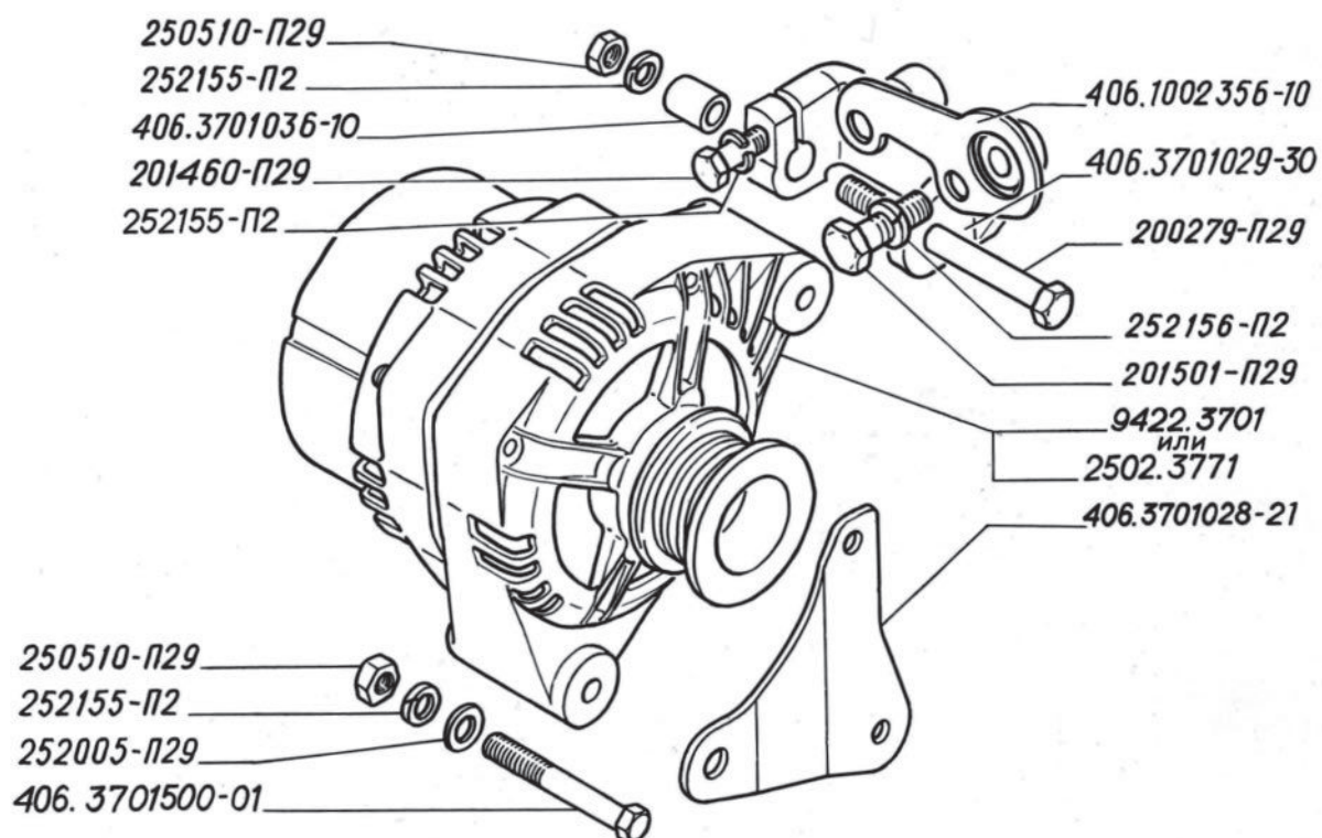
Рис. 72. Генератор двигателей 3М3-406
