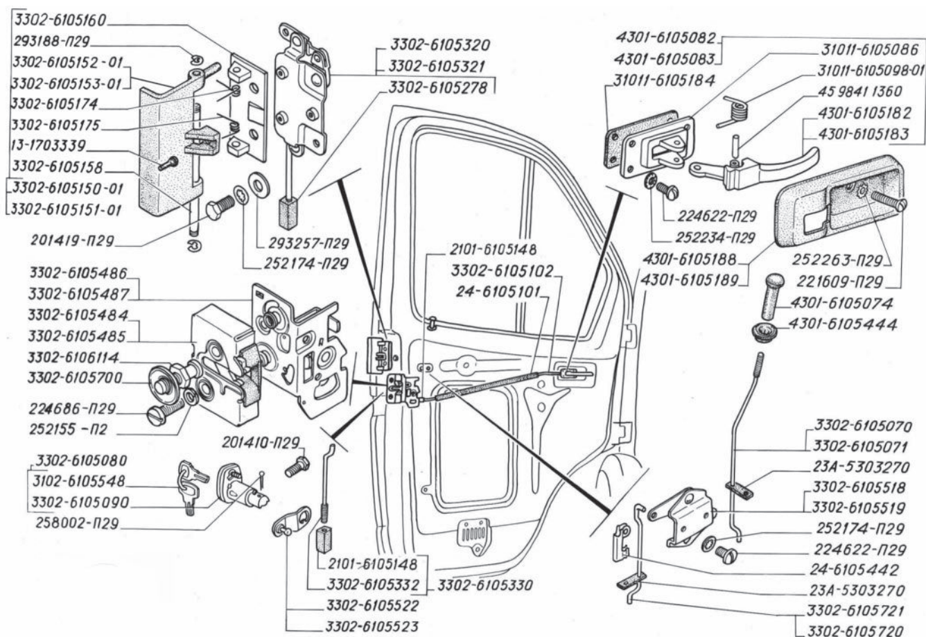
Рис. 105. Замок и ручки дверей кабины (для автомобилей выпуска до февраля 2000 г.)
