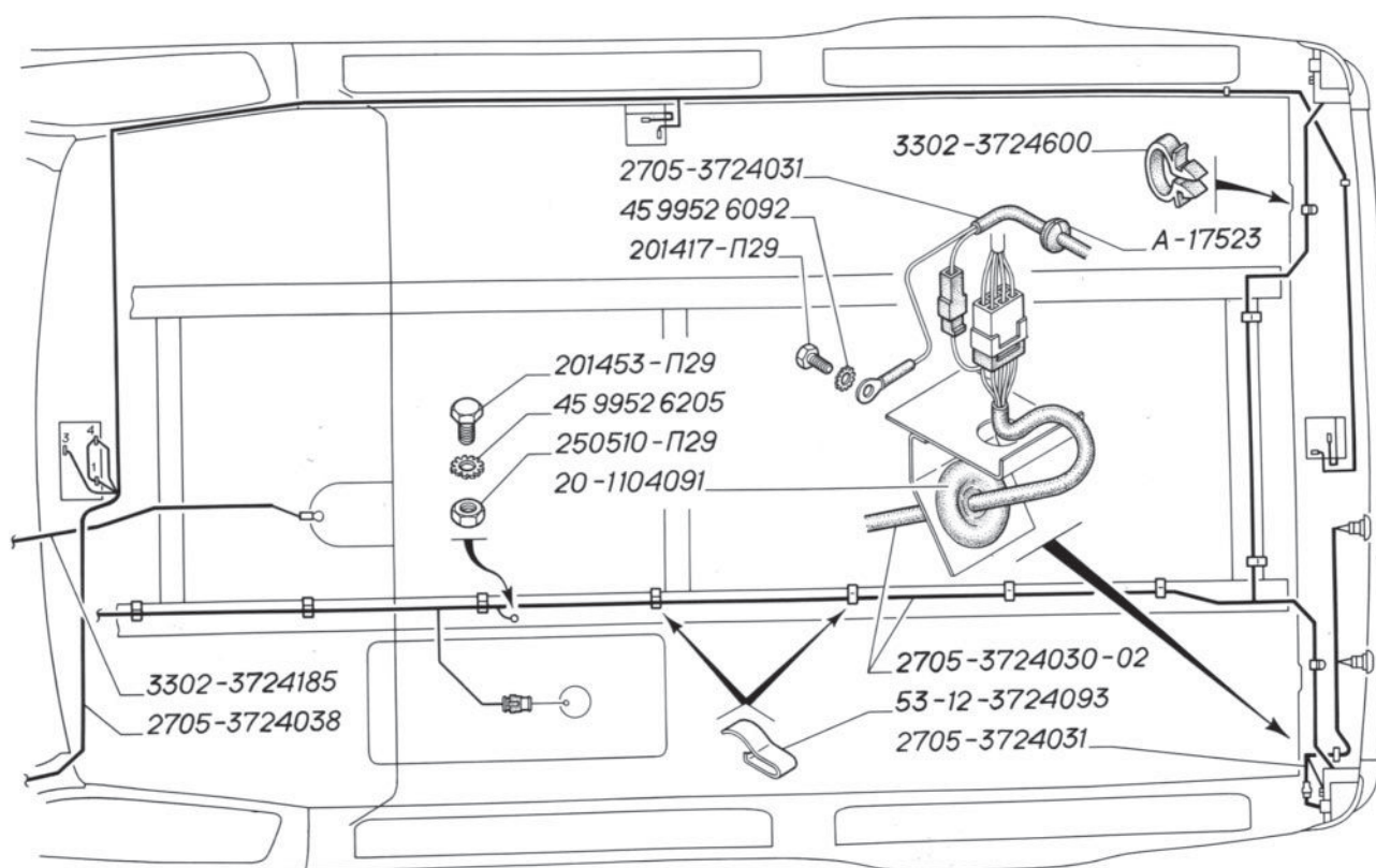
Рис. 81. Электропровода (грузовой отсек)
