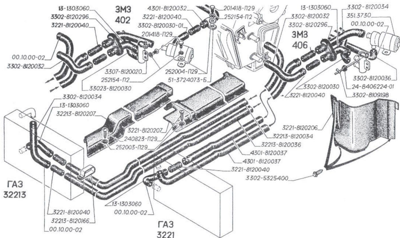
Рис. 30. Трубопроводы отопителей, электронасос (для автобусов выпуска до 2003 г.)
