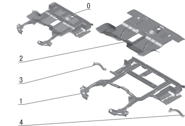
Рис. 8. Каркас с полом передний (3221-5101012-20)
