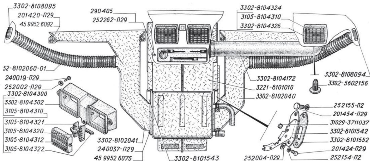
Рис. 117. Отопитель, патрубки обогрева ветрового стекла, воздухопровод и патрубки вентиляции кабины, шланги и патрубки обогрева боковых стекол (для автомобилей выпуска до 2003 г.)
