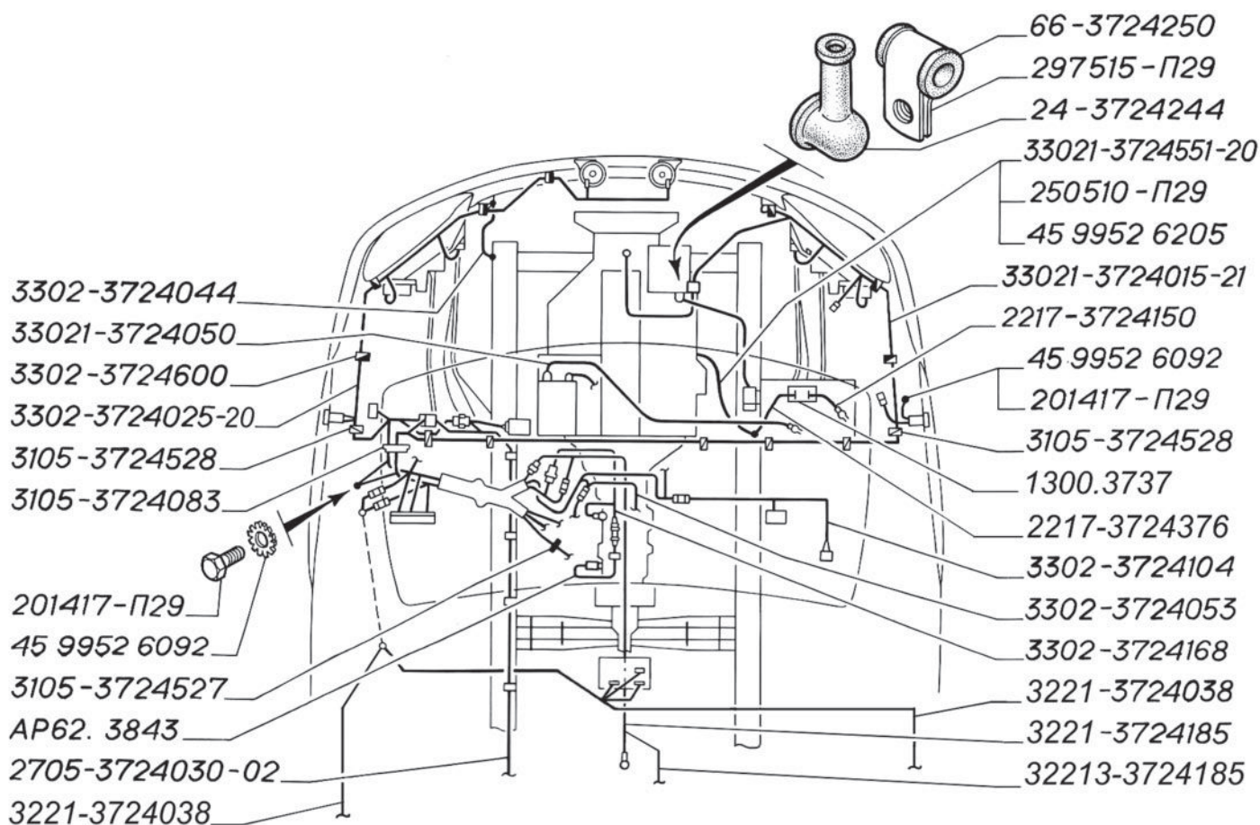
Рис. 10. Установка электропроводов в моторном отсеке и кабине (для автобусов с двигателями 3МЗ-402 и УМЗ-4215)
