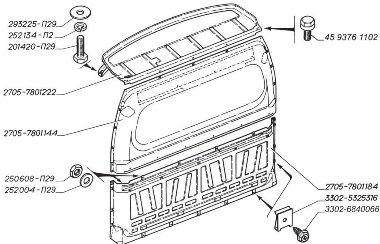
Рис. 116. Перегородка кузова
