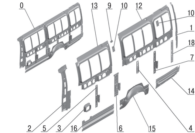
Рис. 139. Каркас левой боковины (3221-5401051)
