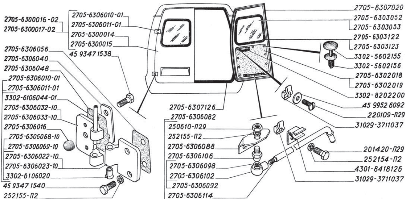
Рис. 108. Двери задка, навеска дверей, обивка, поручень, стекла, кант проема дверей задка
