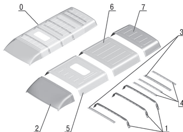
Рис. 425. Крыша (3221-5700012-10)
